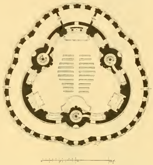
Fig. 56. Dreifaltigkeitskapelle bei Waldsassen. Grundriss.
